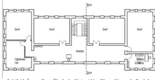
Şekil 13. İsmet Paşa İlkokulu Birinci Kat Planı (Kaynak: Parlak, 2016; Eroğlu 2001: 221)
