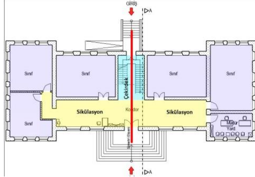
Şekil 12. İsmet Paşa İlkokulu Plan Şeması (Kaynak: Parlak, 2016; Eroğlu, 2001: 220)
