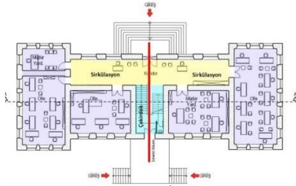
Şekil 7 Hakimiyet-i Milliye İlkokulu Plan Şeması (Kaynak: Parlak, 2016; İl Milli Eğitim Müdürlüğü Arşivi)
