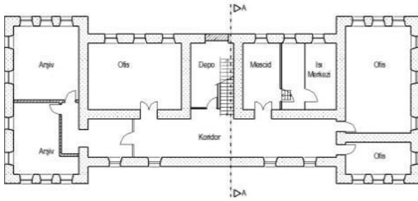
Şekil 4. Gazi Mustafa Kemal İlkokulu Bodrum Kat Planı (Kaynak: Parlak, 2016; Kültür ve Tabiat Varlıklarını Koruma Kurulu Arşivi)
