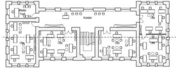
Şekil 8. Hakimiyet-i Milliye İlkokulu Birinci Kat Planı (Kaynak: Parlak, 2016; İl Milli Eğitim Müdürlüğü Arşivi)
