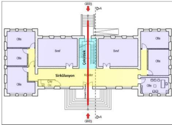
Şekil 2. Gazi Mustafa Kemal İlkokulu Plan Şeması (Kaynak: Parlak, 2016; Kültür ve Tabiat Varlıklarını Koruma Kurulu Arşivi)
