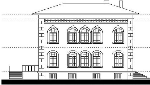
Şekil 11. Hakimiyet-i Milliye Doğu Cephesi
