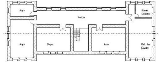
Şekil 9 Hakimiyet-i Milliye İlkokulu Bodrum Kat Planı (Kaynak: Parlak, 2016; İl Milli Eğitim Müdürlüğü Arşivi)
