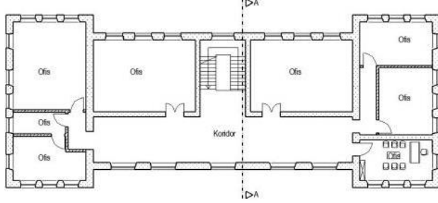
Şekil 3. Gazi Mustafa Kemal İlkokulu Birinci Kat Planı (Kaynak: Parlak, 2016; Kültür ve Tabiat Varlıklarını Koruma Kurulu Arşivi)
