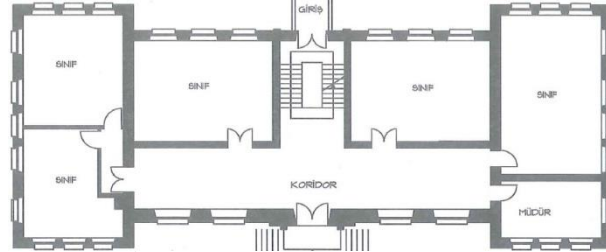
Şekil 1. Tip İlkokul Yapısı Zemin Kat Plan Şeması (Kaynak: Erdoğan 2009: 312)
