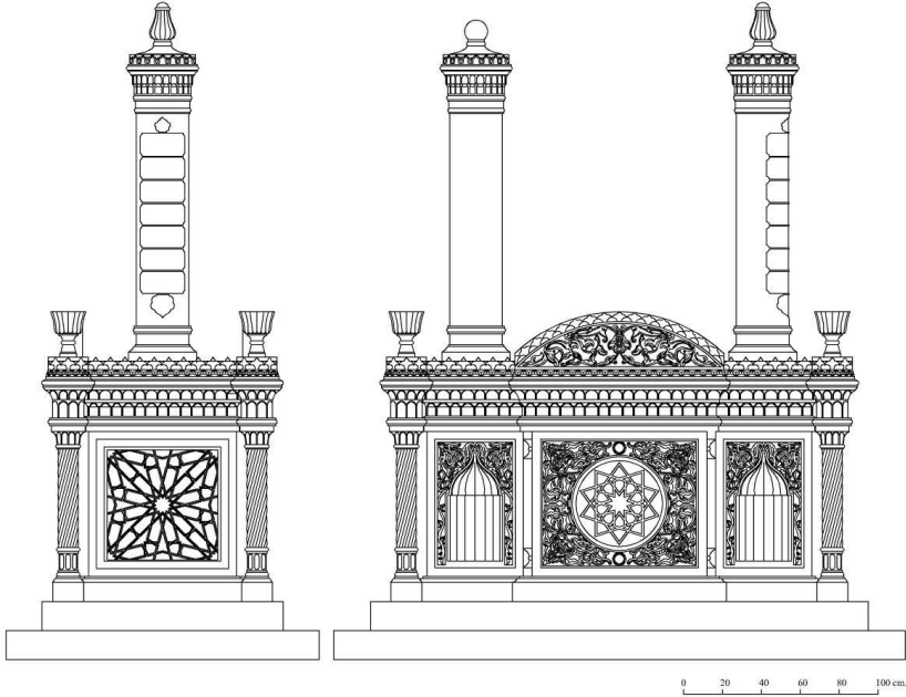
Çizim 5-6. Mehmet Sait Paşa Lahdi ön ve yan cephe görünüşü.
