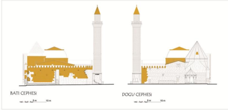
Fot. 14. 1960 onarımı sonrası yapıda görülen değişimler (Vakıflar Arşivinde yer alan rölöve çizimleri kullanılarak yapılmıştır)
