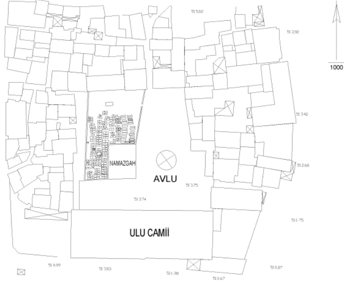
Çizim 1 Urfa Ulu Camii ve Haziresi Vaziyet Planı
